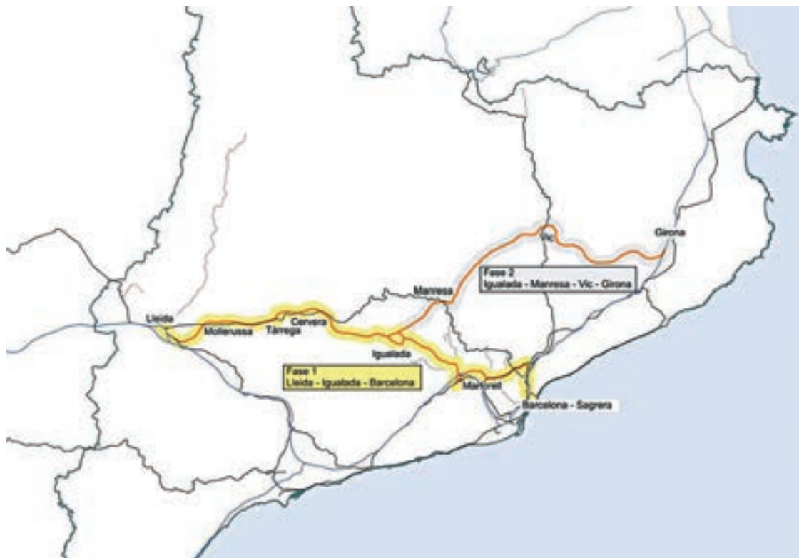
FOTO_ Departament de Territori Recorregut del futur Eix Transversal Ferroviari, amb el ramal que connectarà Igualada amb l'estació de la Sagrera de Barcelona
