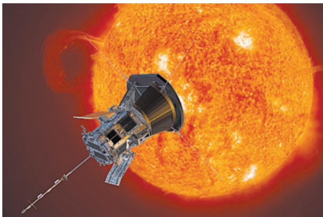
FOTO_NASA La sonda solar Parker s'atansa molt al sol i aportarà dades inèdites
